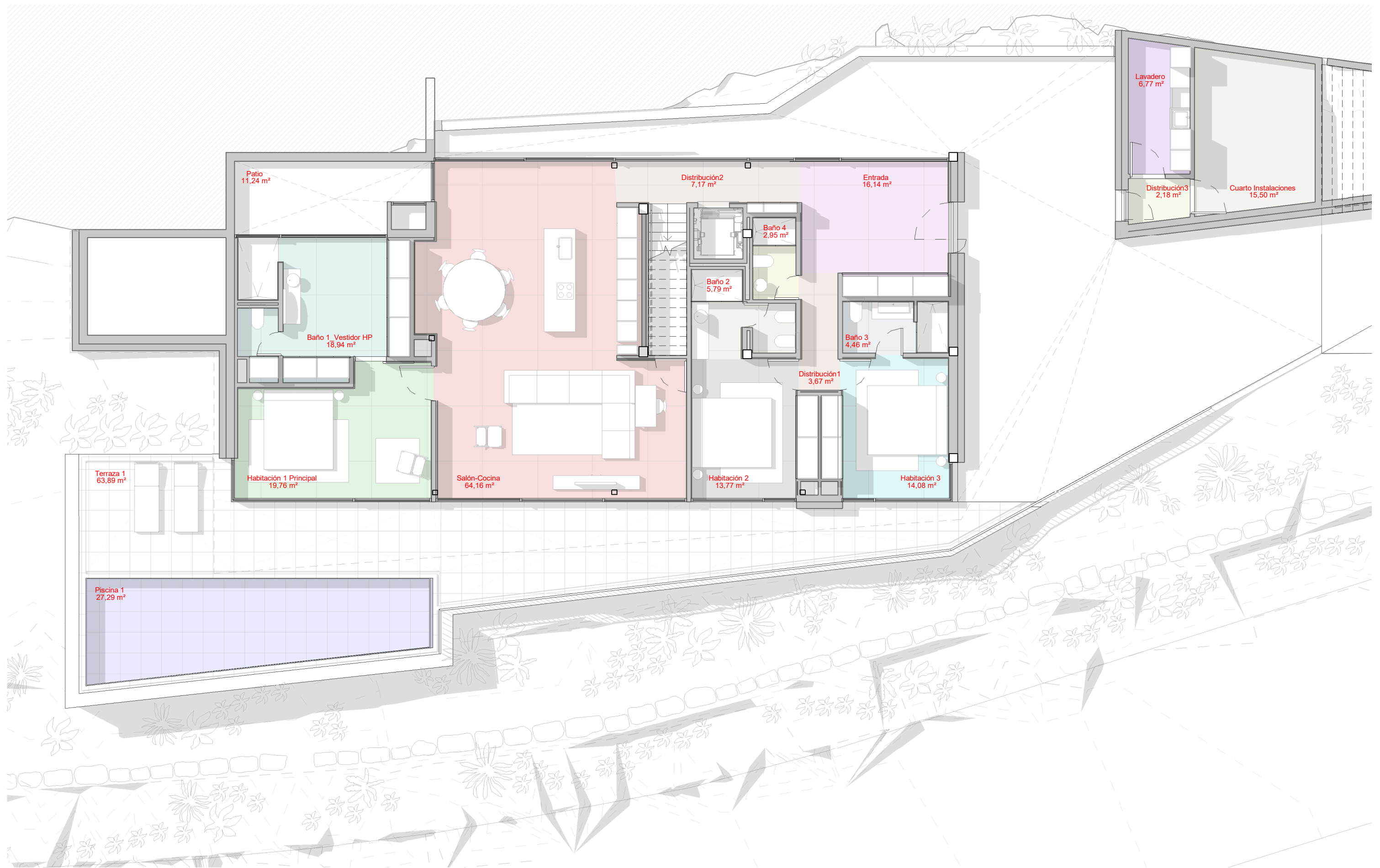
Planta Baja 1 : 100
